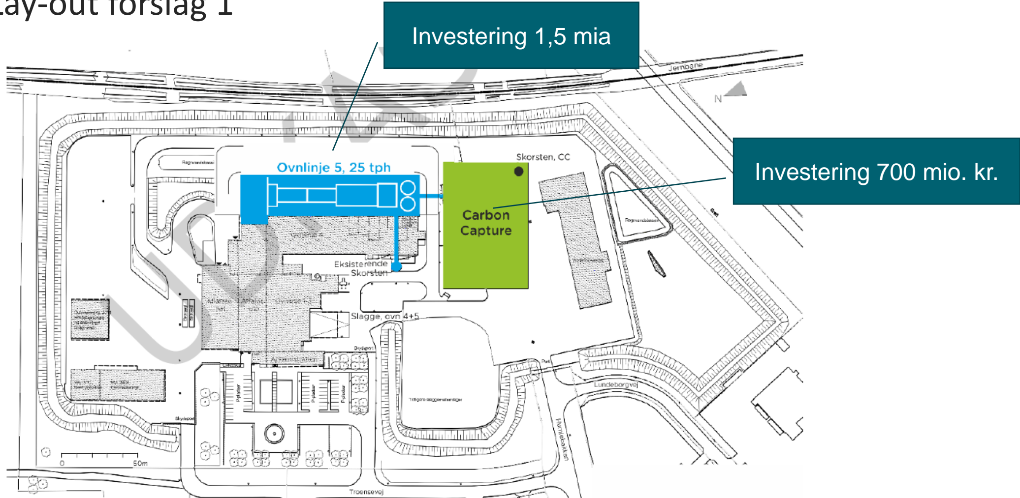
Figur 10 Layoutforslag #1 med placering af en ny ovnlinje 5 ud mod banen.
